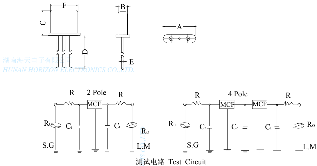
选型尺寸表 Dimensions Table
