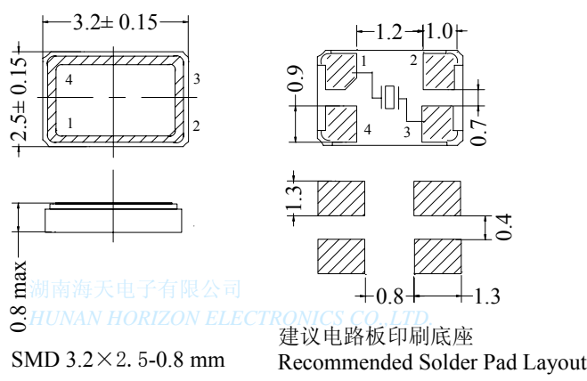
外形尺寸(单位:毫米) Figure and Dimensions(Unit: mm)
